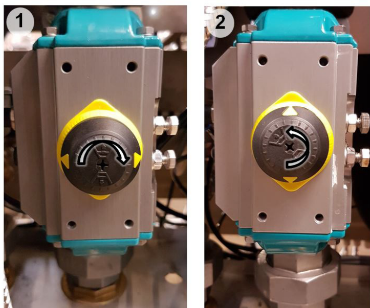
Fig. 0-119 Stillingsindikator ventilaktuator for køling
