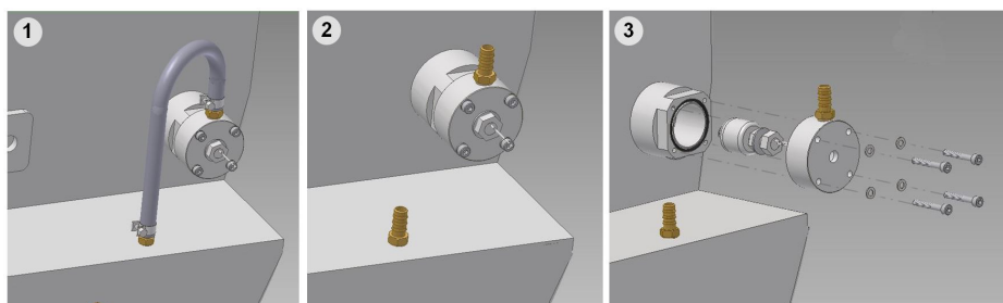
Fig. 0-111 Adskillelse af niveauhus
