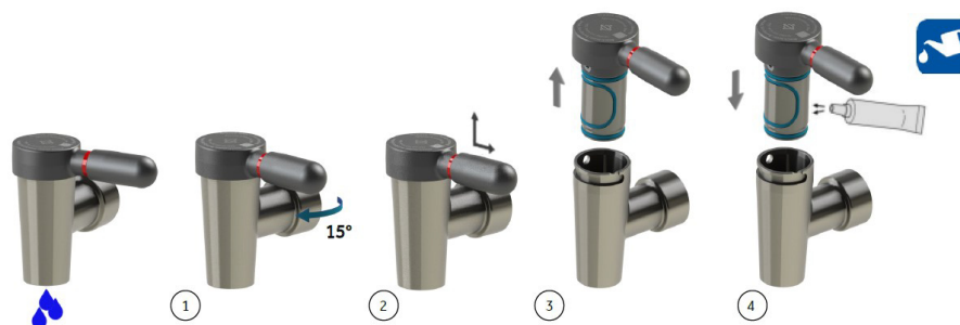
Fig. 0-76 Adskildelse af aftapshane
