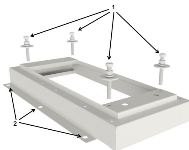
Fig. 0-11 Fixtur
