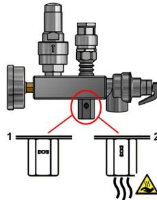
Fig. 0-88 Kuglehane til kontrolmanometer
