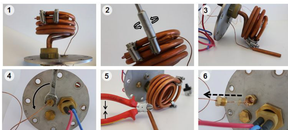
Fig. 0-126 Demontage af tørkogningssikring
