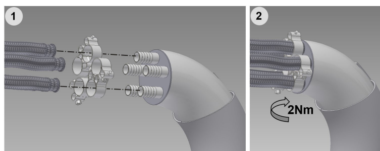
Fig. 0-20 Slanger for kølevand retur 150 - 500 l *
