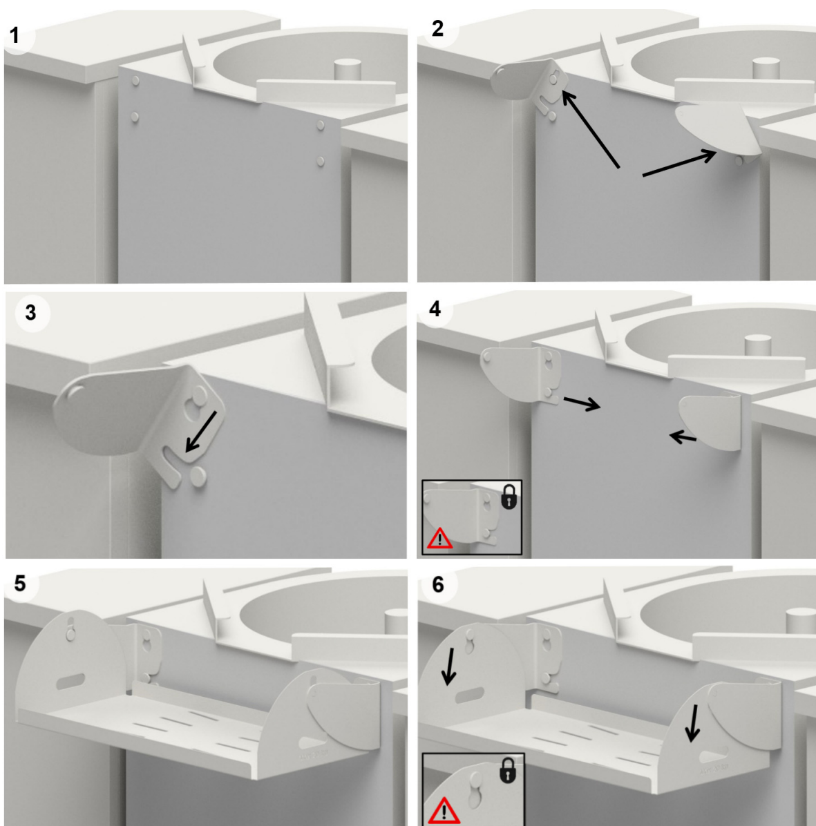
Fig. 0-59 Fastgørelse af kantineholder på gryder med flad front
