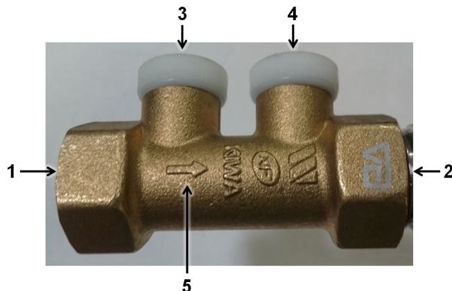
Fig. 0-101 Kontraventil
