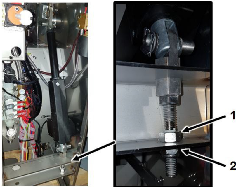
Fig. 0-97 Stående aktuator
