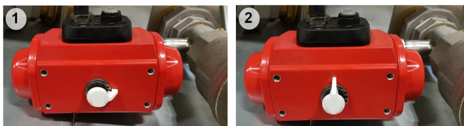
Fig. 0-120 Stillingsindikator ventilaktuator for tømning
