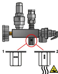
Fig. 0-84 Kuglehane til kontrolmanometer
