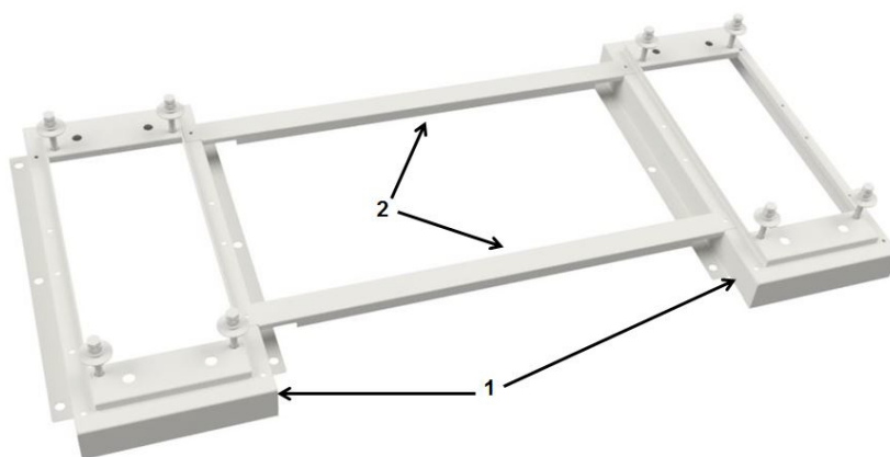
Fig. 0-12 Samlet fixtur monteret med afstandsskinner
