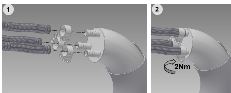
Fig. 0-19 Slanger for kølevand frem for 150 til 500 l *
