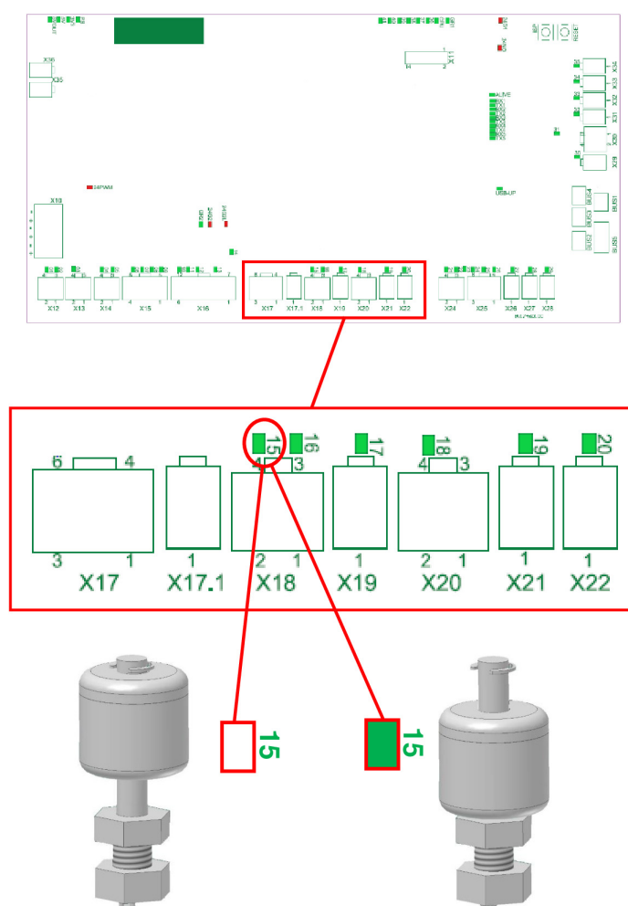
Fig. 0-116 Niveaufbryderens statusindikation på AutoChef 82 og AutoChef 86 printkortets bagside.
