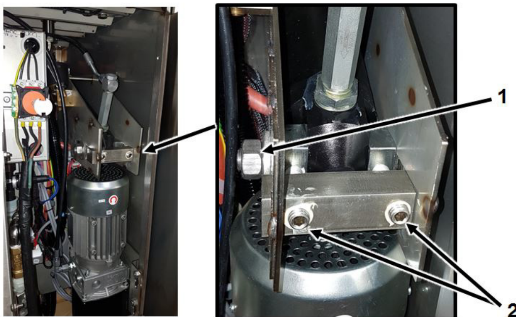
Fig. 0-99 Hydraulik
