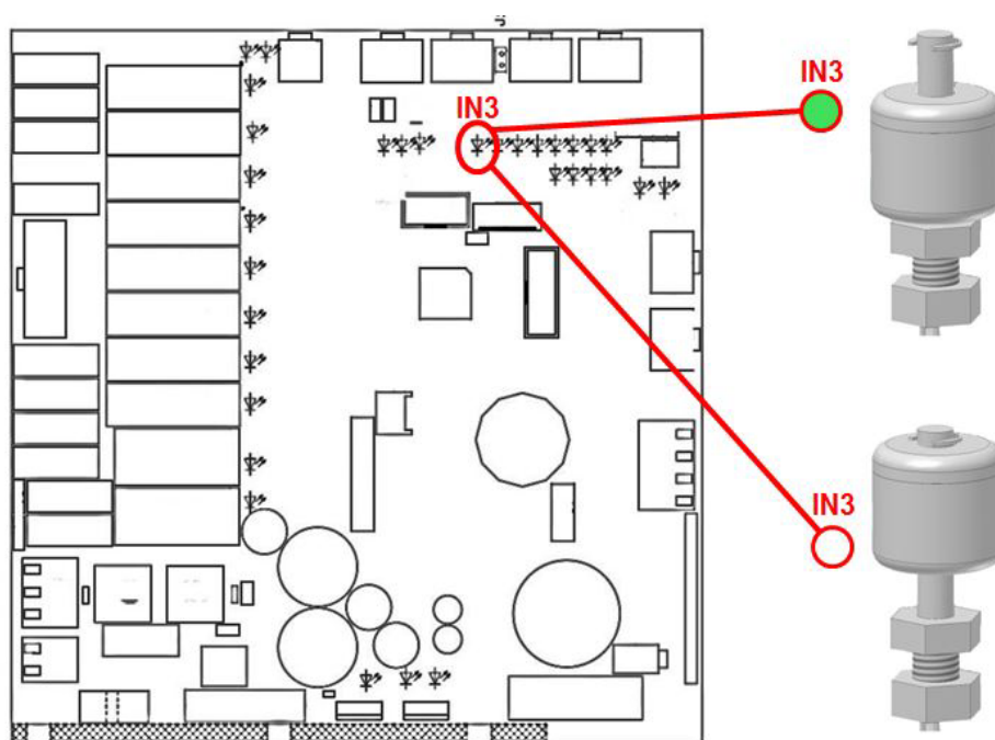
Fig. 0-113 Niveaufbryderens statusindikation på printkortets bagside.
