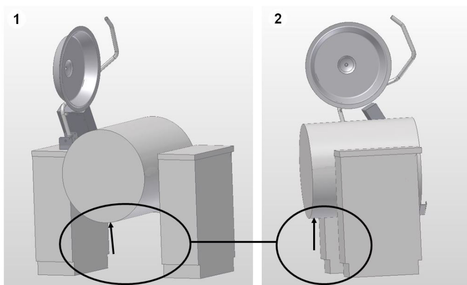
Fig. 0-80 Punkt for understøtning ved kippet gryde
