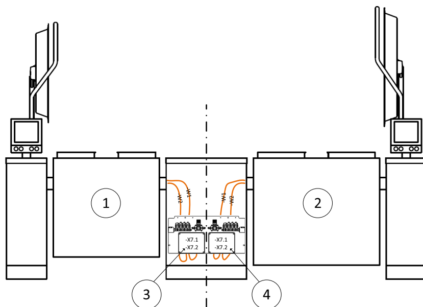
Fig. 0-16 Elektrisk sammenbygning af gryder til direkte damp og/eller isvandskøling
