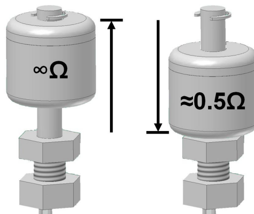
Fig. 0-109 Niveaufbryderens funktionalitet
