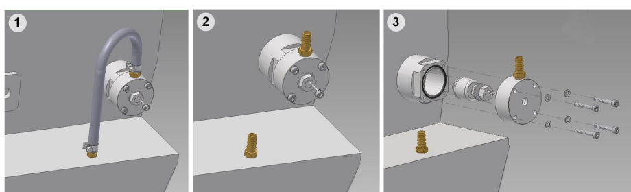
Fig. 0-117 Adskillelse af niveauhus
