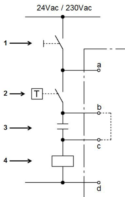
Fig. 0-7 Koblingsprincip for effektregulering
