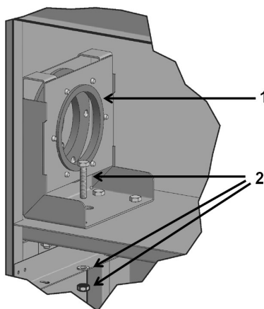
Fig. 0-14 Støtteleje
