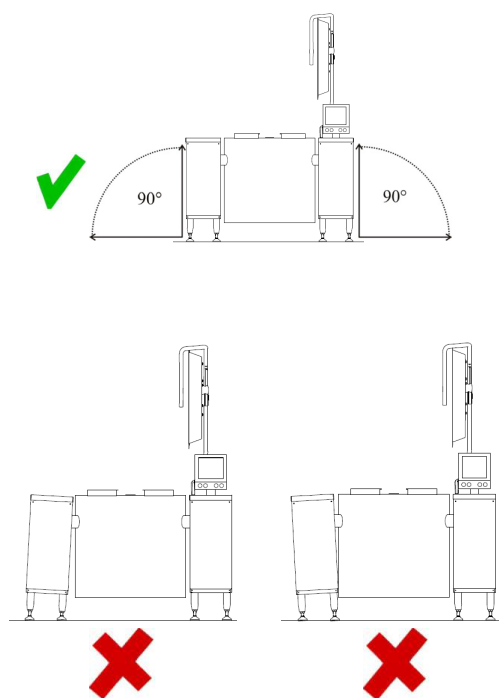
Fig. 0-8 Gryden i lod og vater fra fronten
