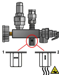
Fig. 0-86 Kuglehane til kontrolmanometer
