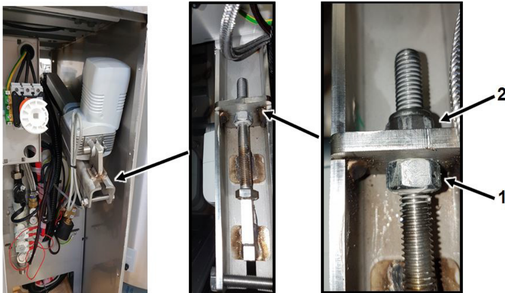
Fig. 0-98 Liggende aktuator
