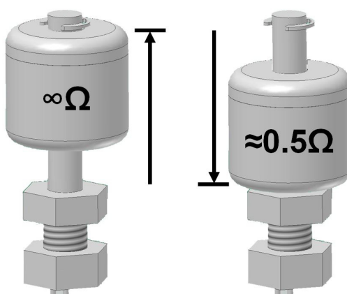
Fig. 0-112 Niveaufbryderens funktionalitet
