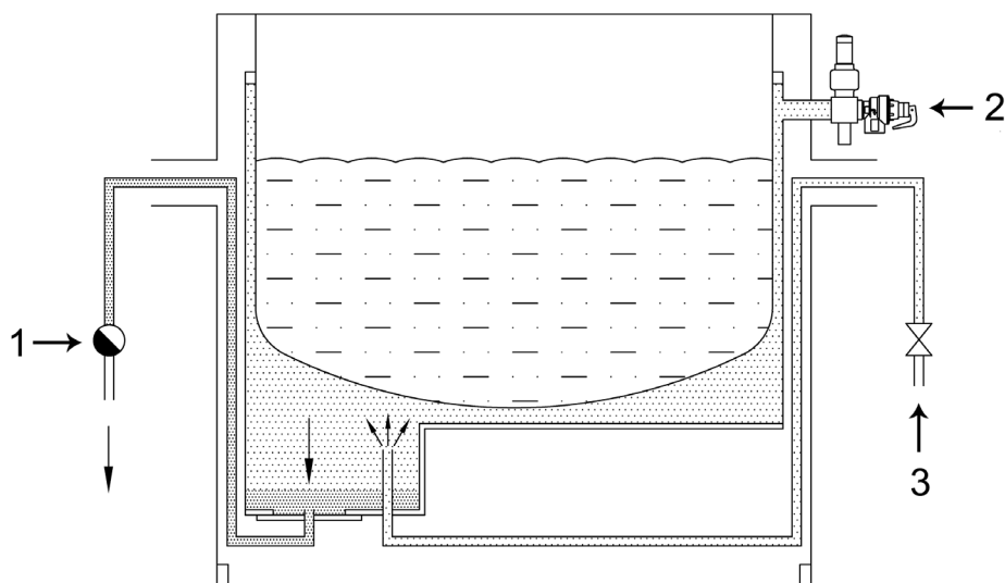
Fig. 0-83 Princip damp-opvarmet gryde
