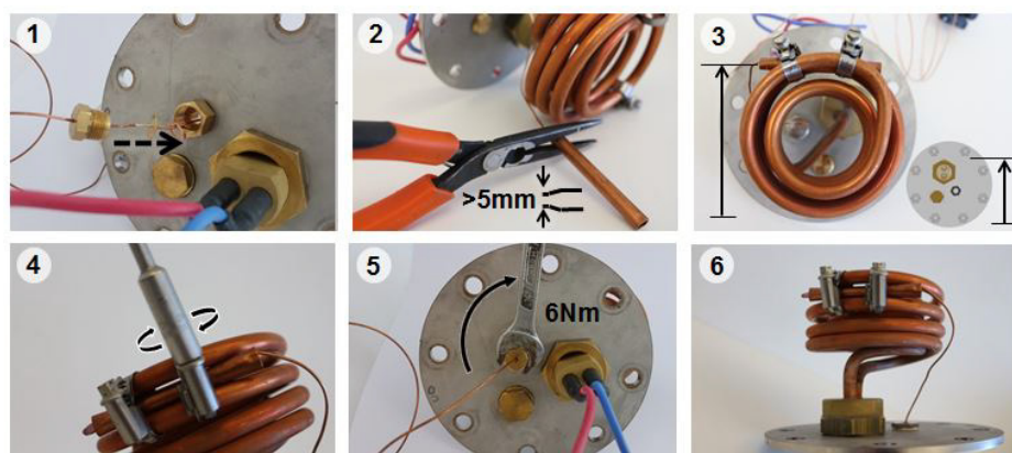
Fig. 0-127 Montage af tørkogningssikring
