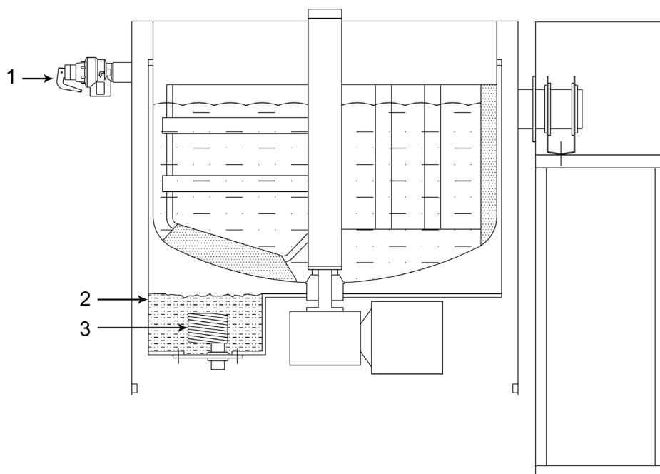
Fig. 0-82 Princip el-opvarmet gryde
