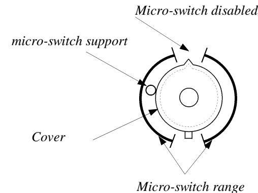
FIG.n°8 - Jug position
