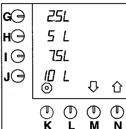
Fig. 23 Standardforvalgknapper
