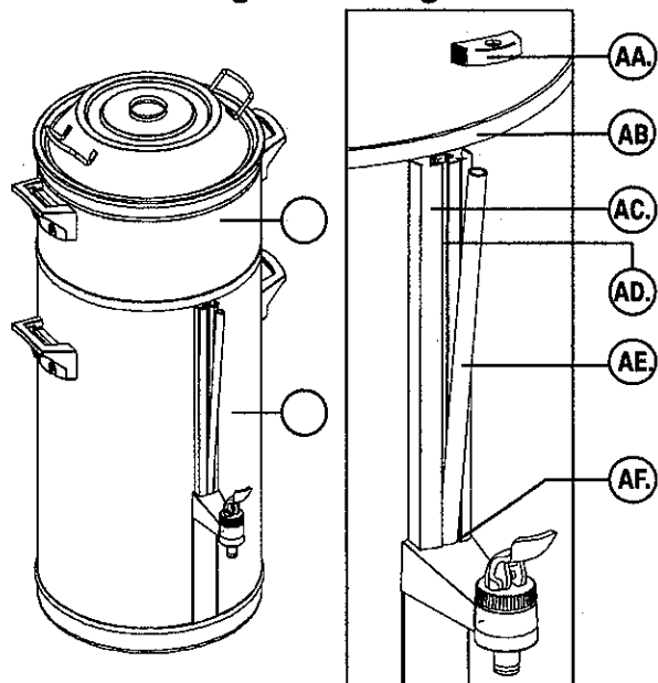
Fig. 8 Anbringelse af kontrolglassets låg
