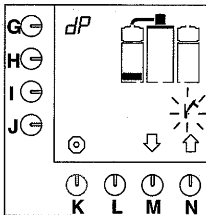
Fig. 17 Kaffebryggerens første niveau af afkalkningsprogrammet
