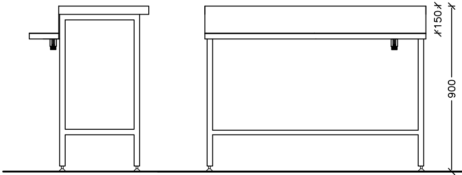
RS bord til kaffemaskiner 10L/20L/40L med nedsænket drypbakke.
