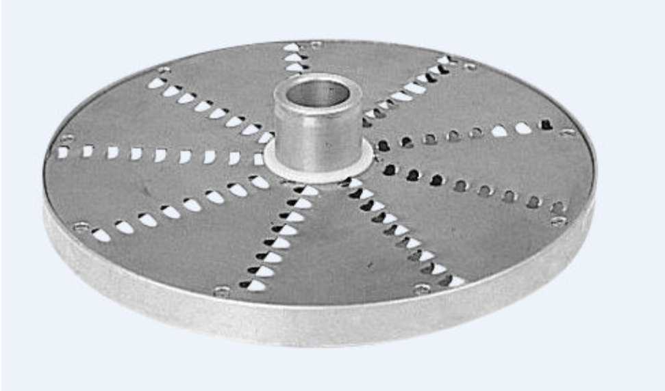
Råkostskive 6 mm Udført i rustfrit stål til RG 3001 OB/71225702
