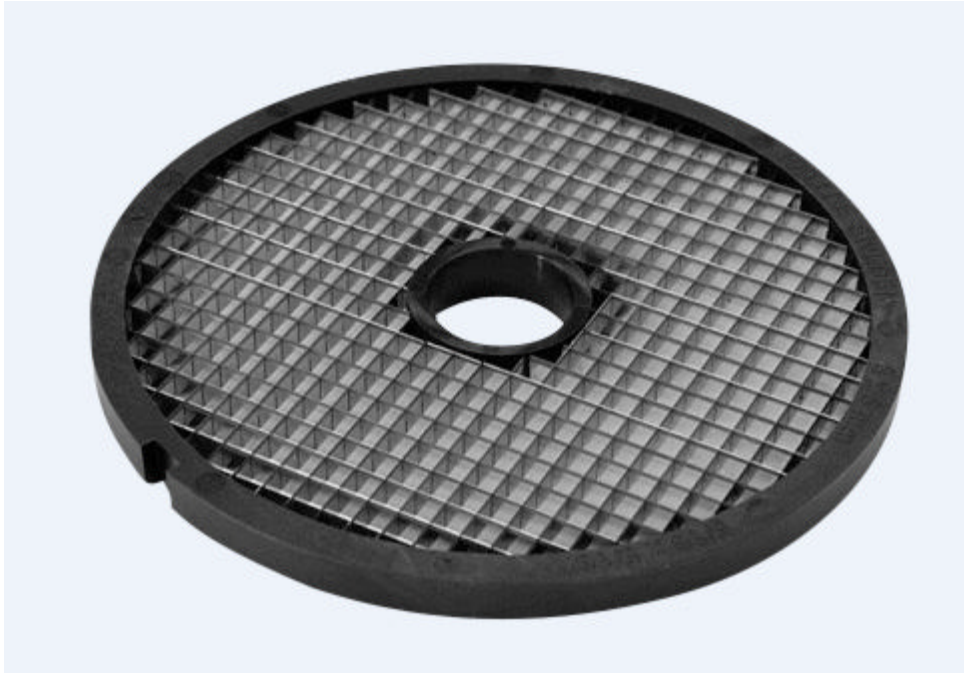
Terningsgitter 10 x 10 mm Udført i rustfri stål og plast Til RG 50 OB/71229701
